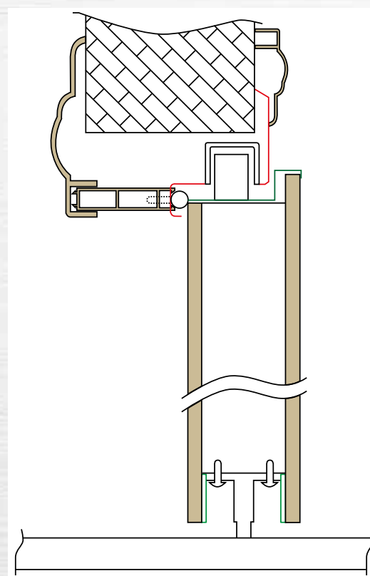
Κάθετη τομή / Vertical section
