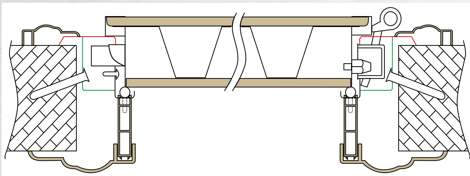
Σχέδιο συναρμολόγησης περβαζιών και επενδύσεων ΑΛΟΥΜΙΝΙΟΥ σε πόρτα. Οριζόντια τομή. Typical assembly of trims and leaf's covers on door. Horizontal section.
