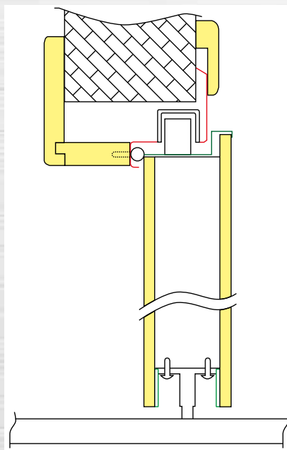
Κάθετη τομή / Vertical section
